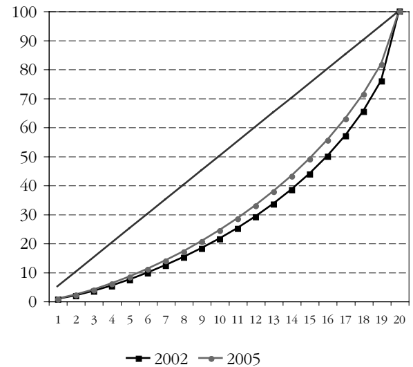
Grafik.22 - Lorenz Eğrisi
